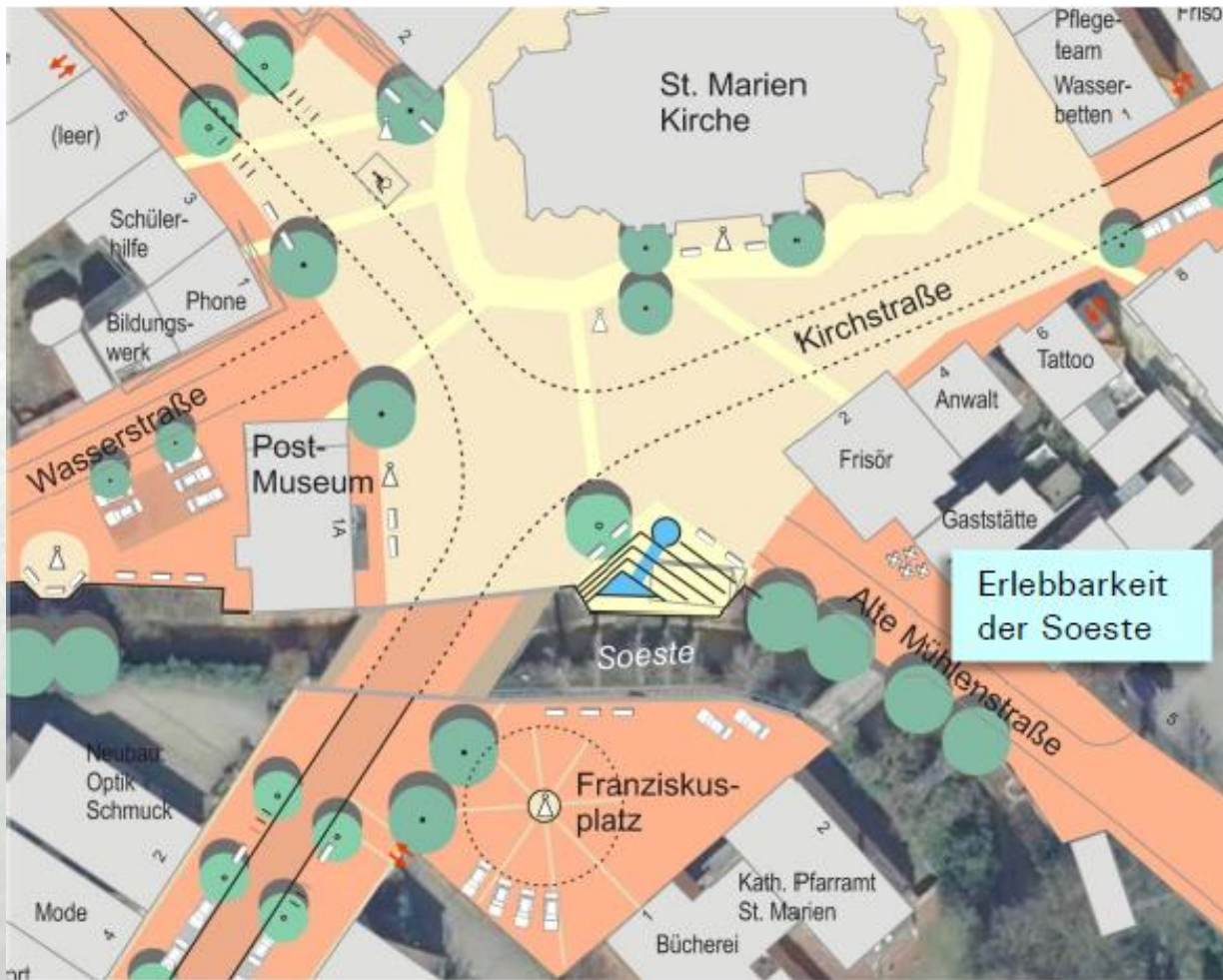
Zentraler Knotenpunkt – Einmündung/Shared Space, helle Fahrbahn, gestalterische Einbeziehung des Kirchplatzes (Variante 4) (empfohlen)
